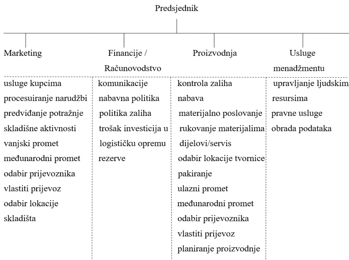
Slika 1. Organizacijska struktura integralne logistike
