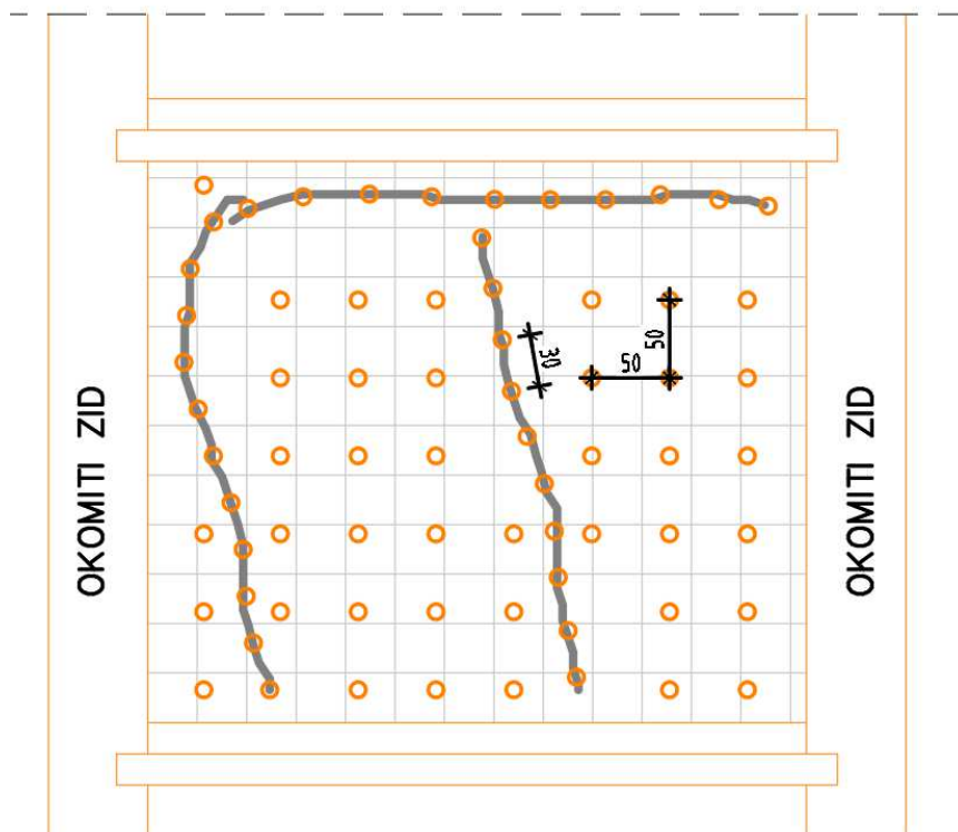
Slika 42. Prikaz injektiranja zida
