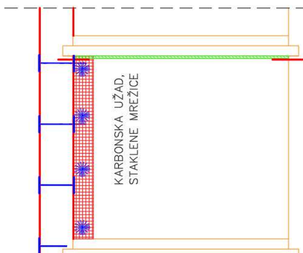
Slika 43. Presjek kroz vanjski zid
