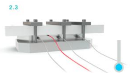
Slika 5.4 Pozicioniranje obratka i primjena adhezije [34]
