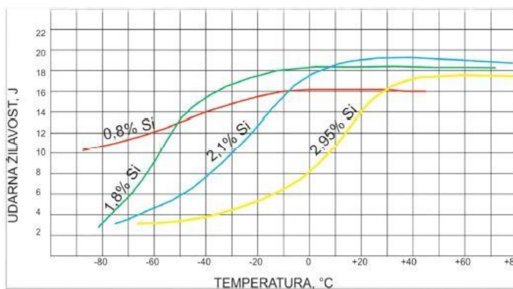
Slika 2.6 Odnos temperature na udarnu žilavost pri različitim udjelima silicija [13]
