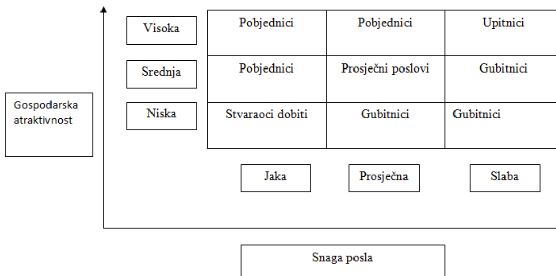
Slika 7. GE matrica
