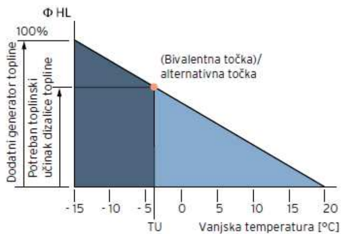
Slika 3.3 Dijagram potrebnog toplinskog učinka dizalice topline kod bivalentno alternativnog načina rada [9]
