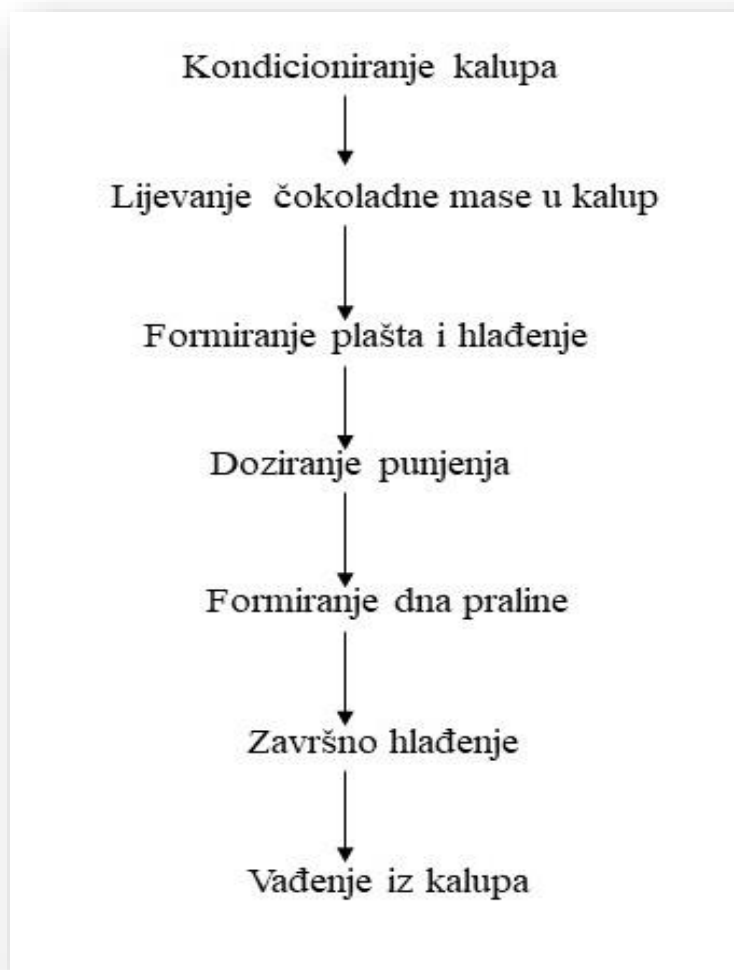
Slika 3: Shema konvencionalne proizvodnje čokoladnih pralina (prema Becket, 2008)
