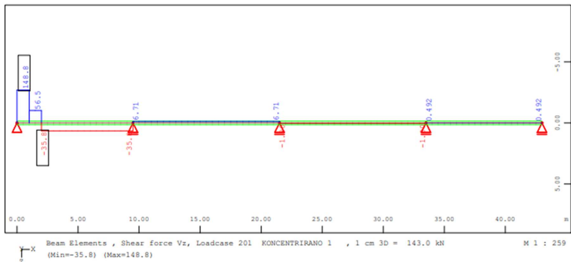
Slika 14. Moment My i poprečne sile Vz od koncentriranih sila kotača na početku prvog polja
