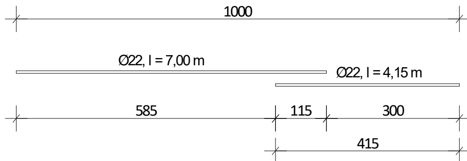
Slika 21. Glavna uzdužna armatura polja 1-4
