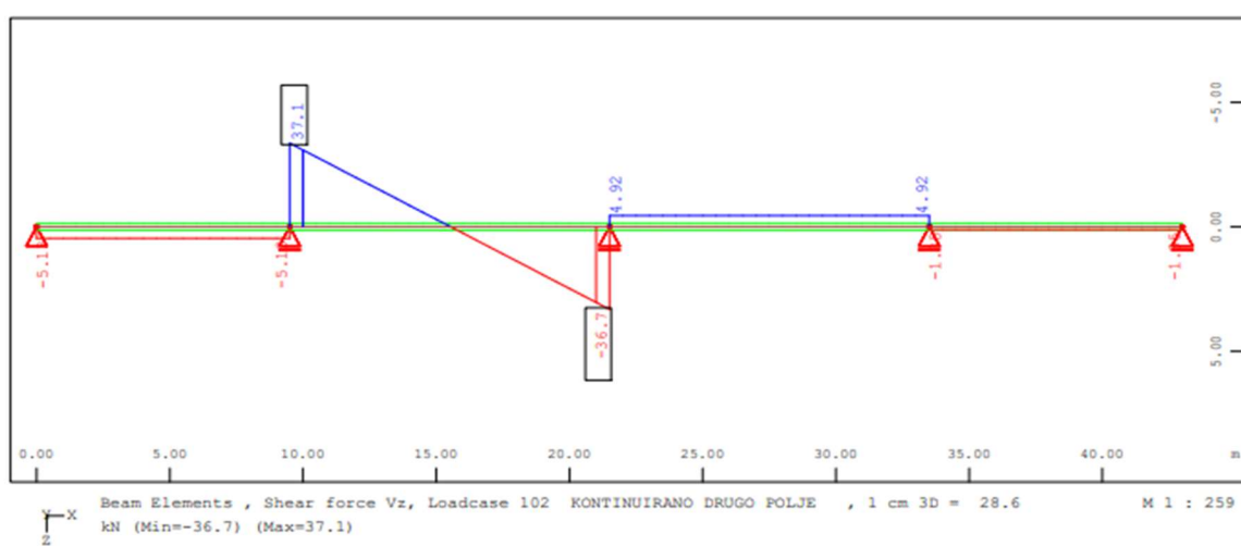
Slika 11. Moment My i poprečne sile Vz od korisnog opterećenja u drugom polju
