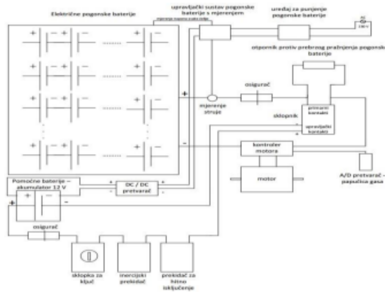
Slika 3.2. Blok shema
