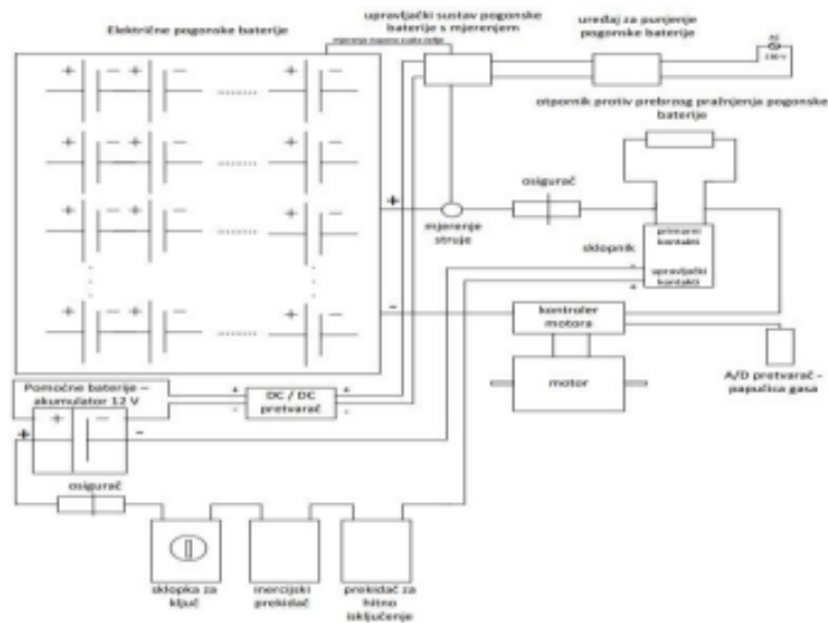
Slika 3.2. Blok shema
