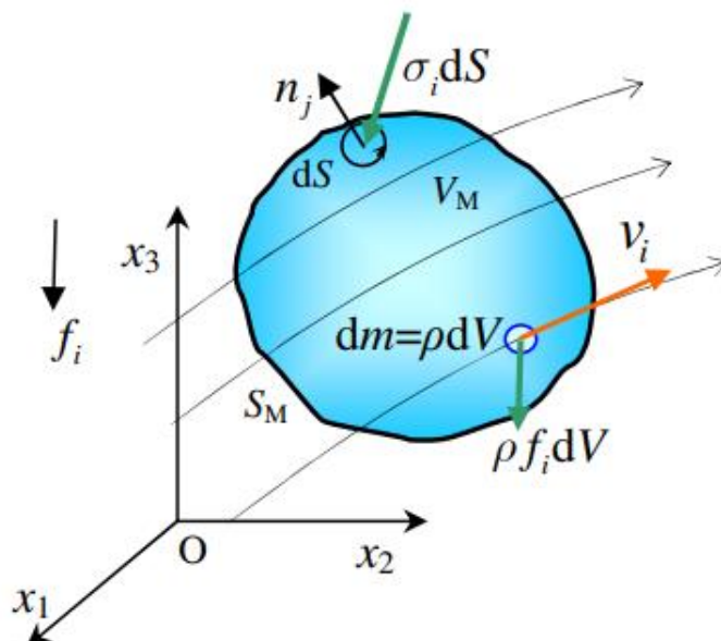
Slika 16. Materijalni volumen [3]
