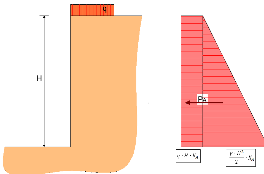
Slika 3.3. Utjecaj dodatnog opterećenja na aktivno naprezanje.
