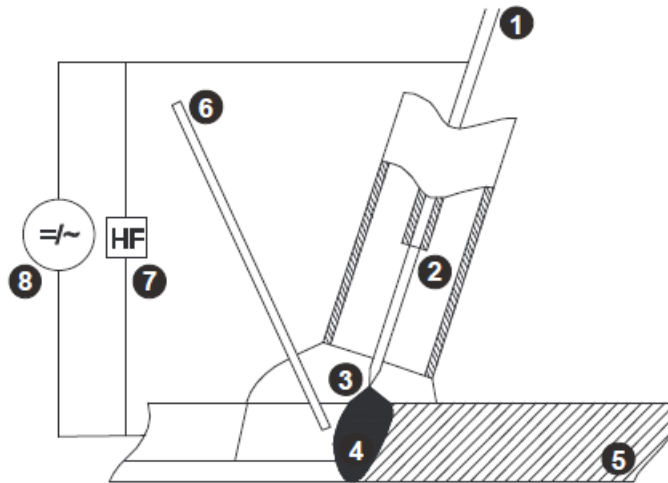
Slika 6. Shematski prikaz procesa TIG zavarivanja 1 – netaljiva elektroda; 2 – sapnica gorionika; 3 – električni luk; 4 – rastaljeni materijal; 5 – osnovni materijal; 6 – dodatni materijal; 7 – visokofrekventni generator, 8 – izvor struje
