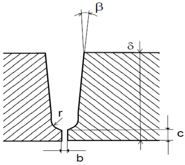
Slika 15. Sučioni U-spoj [37]
