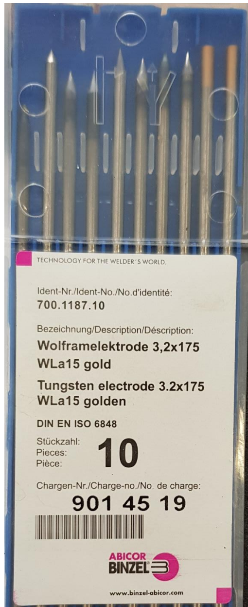
Slika 39. Volframove elektrode
