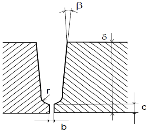
Slika 15. Sučioni U-spoj [37]
