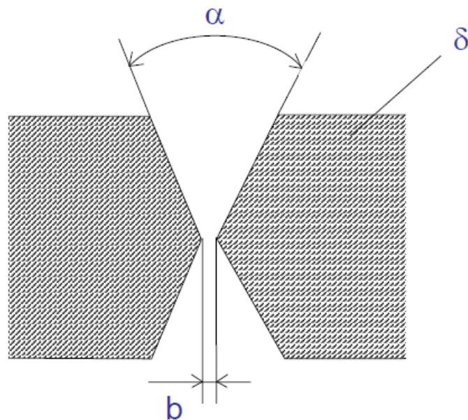
Slika 14. Sučeoni X-spoj [37]
