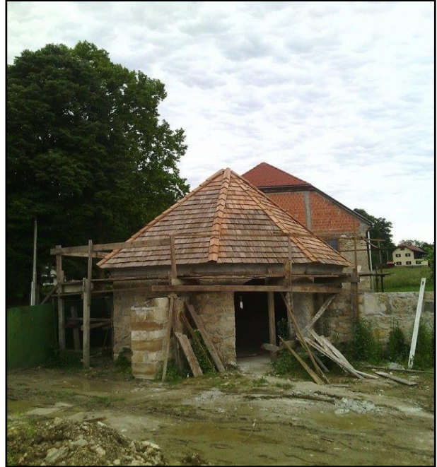
Slika 105. Postava šindre na krovšte kule
