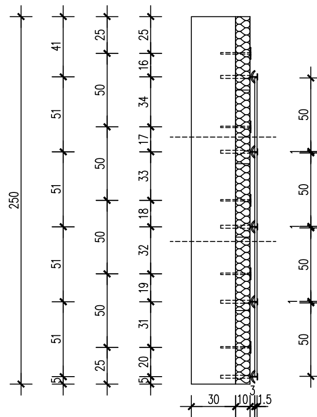
PRESJEK
