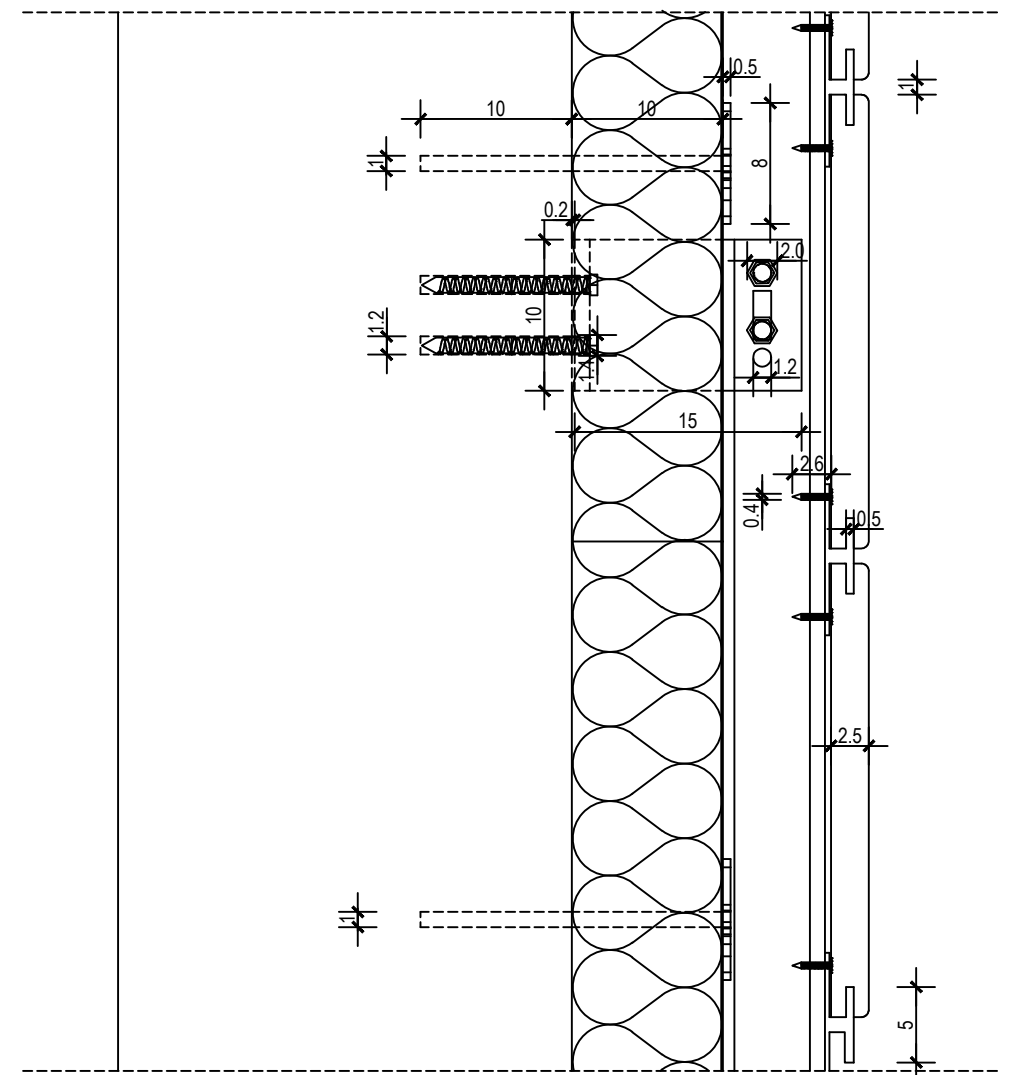
PRESJEK DETALJ 1:5
