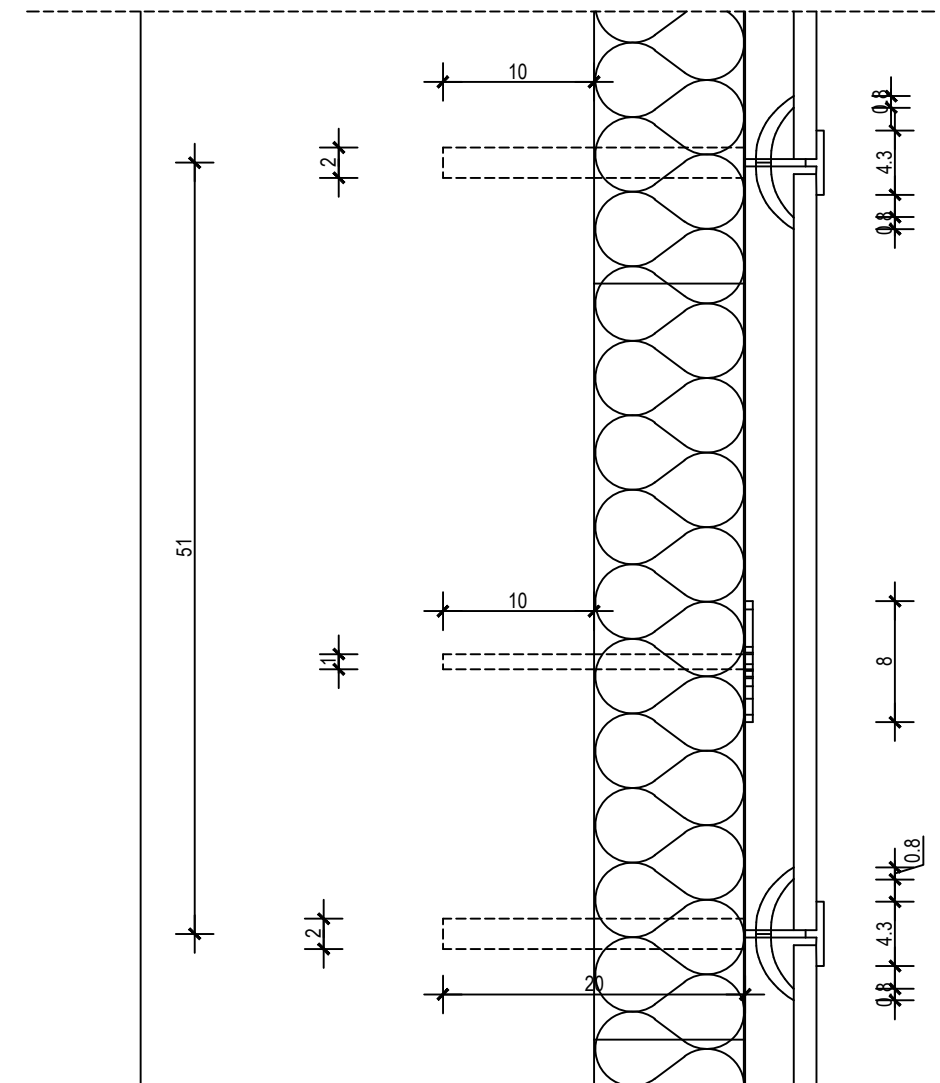
PRESJEK DETALJ 1:5
