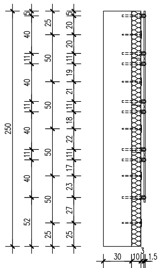
TLOCRT
