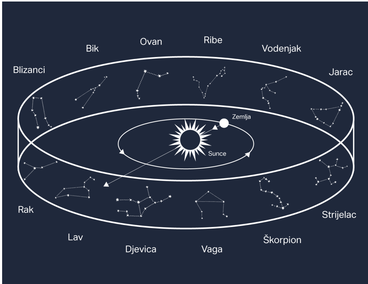
Slika 1.1. Prividno kretanje Sunca kroz sazviježđa gledano sa Zemlje
