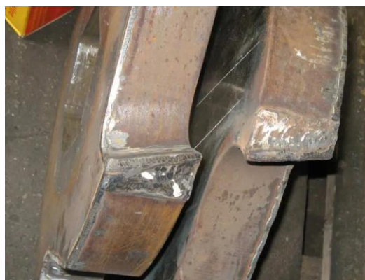
Slika 25. Navareni noževi za mljevenje otpada. [18]
