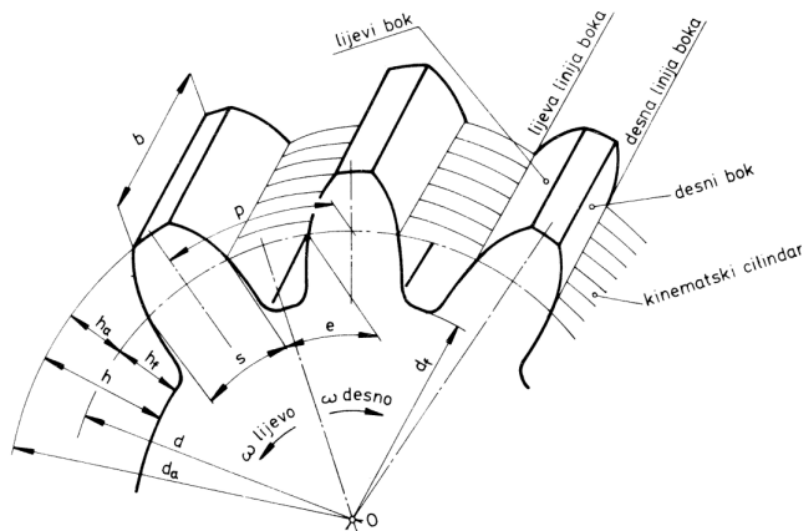
Slika 3.2 Dimenzije zupčanika
