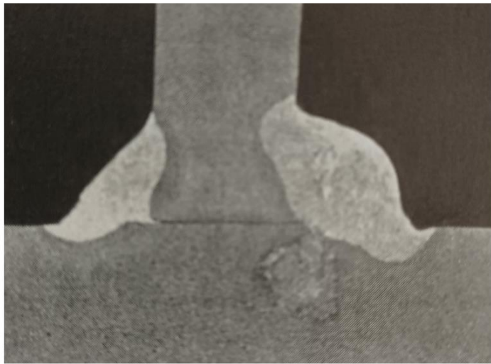
Slika 3.12. Pogreške oblika zavora – ugorine i ispupčenost kutnog zavora [29]
