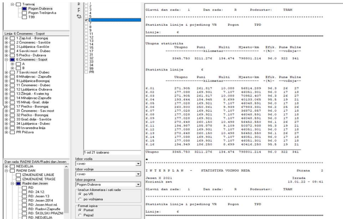
Slika 21: Statistika linije 6;
