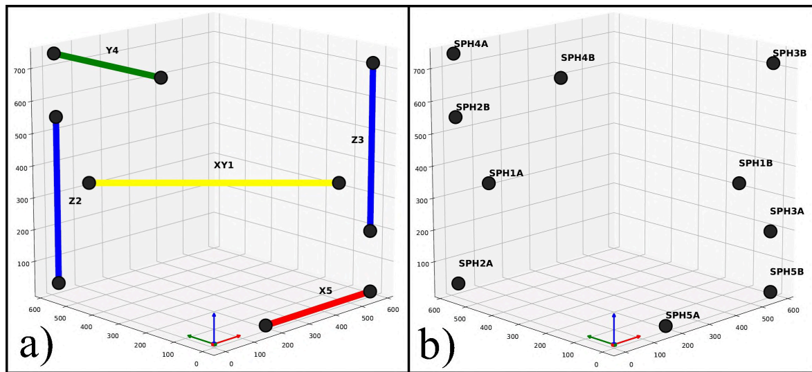
Slika 28: Mjerni volumen: a) Raspored referentnih objekata, b) Raspored sfera [40]
