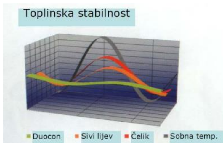
Slika 4 Toplinska stabilnost [10]
