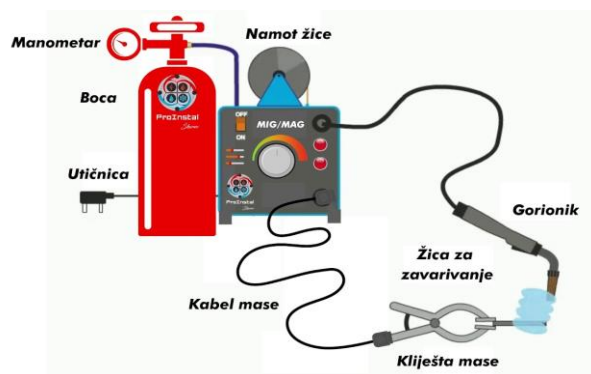
Slika 2.1 Oprema za MIG zavarivanje [4]
