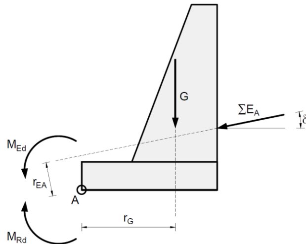
Slika 4.6 Prikaz djelujućih sila kod proračuna potpornog zida na prevrtanje
