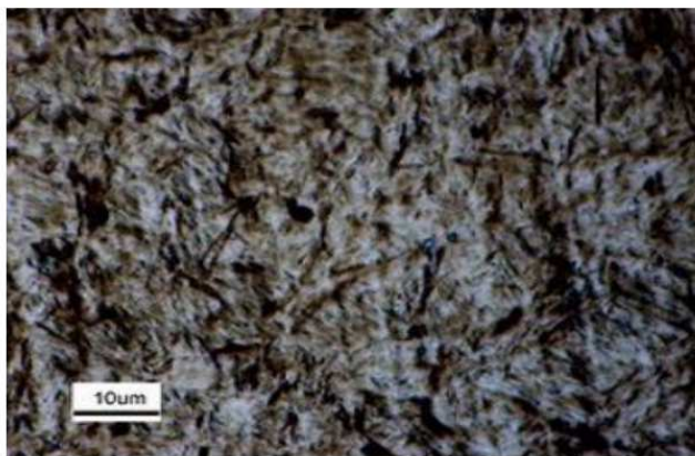
Slika 22. Mikrostruktura martenzitnih nehrđajućih čelika [4]
