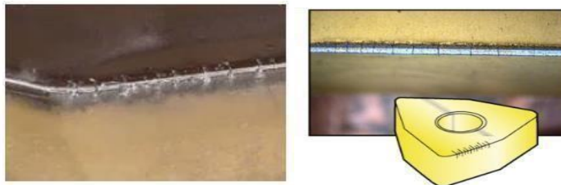
Slika 9.21 Toplinske pukotine [10]
