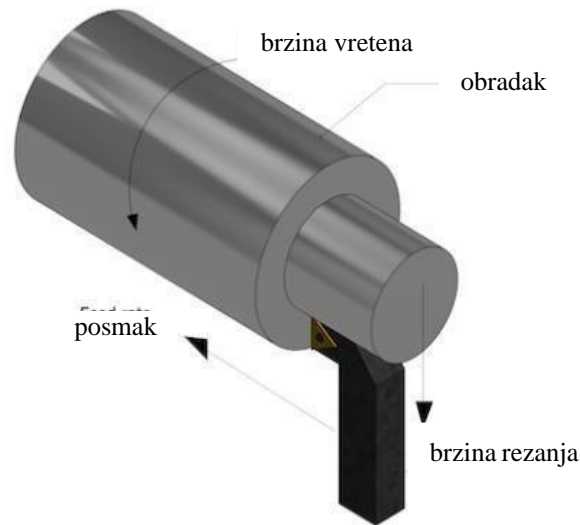
Slika 11.3 Prikaz odnosa brzine rezanja i brzine vretena [24]
