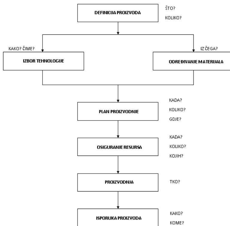
Slika 2.1 Aktivnosti pripreme proizvodnje [2]
