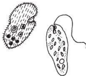
Slika 32. Protozoe [32]
