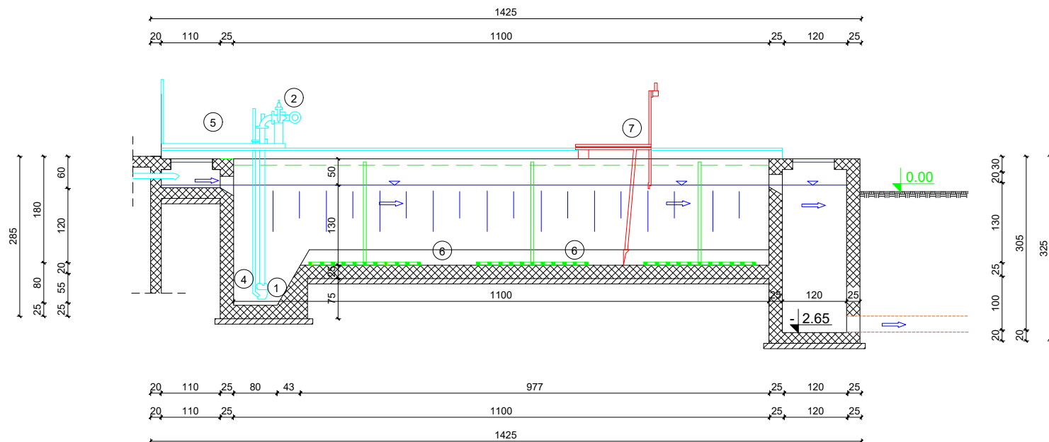
Presjek A-A (uzdužni presjek)
