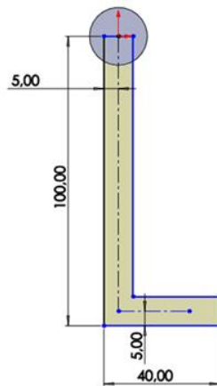
Slika 3.52 Skica igle za orijentiranje čepova
