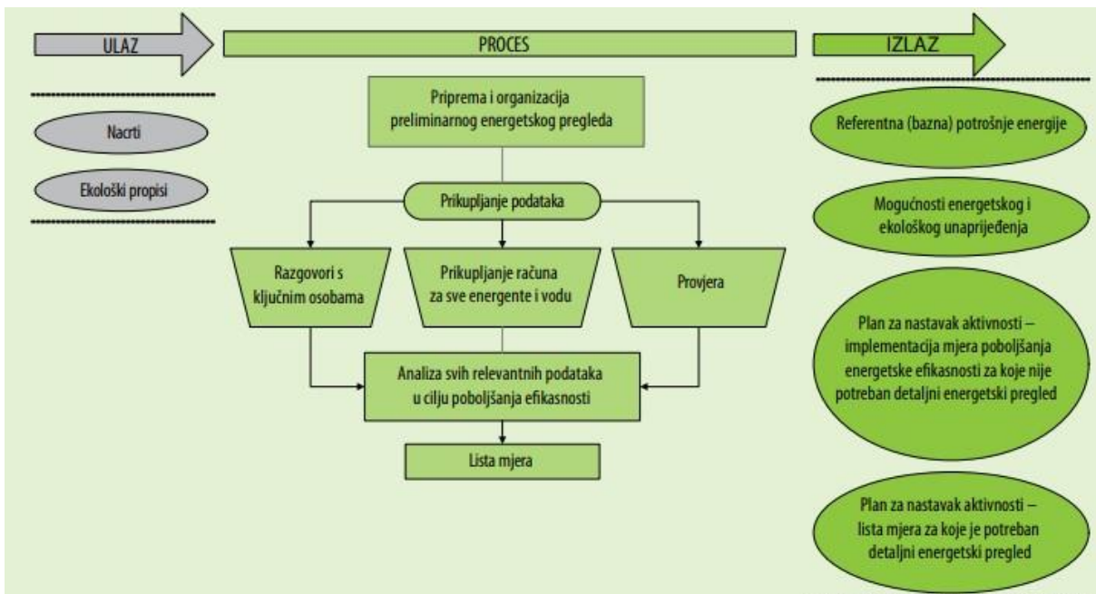
Slika 8- Shema općeg energetske pregleda [23]
