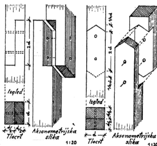
Slika 18. Ravno preklapanje s ravnim sudaranjem (lijevo) i ravno preklapanje s trobridnim sudaranjem (desno) [1]
