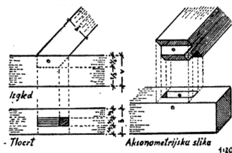
Slika 32. Učepjenje skraćenim otupljenim čepom [1]
