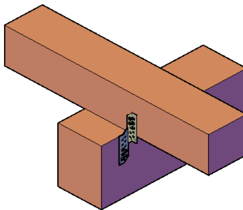
Slika 93. Spoj vezne grede i podrožnice [22,23]
