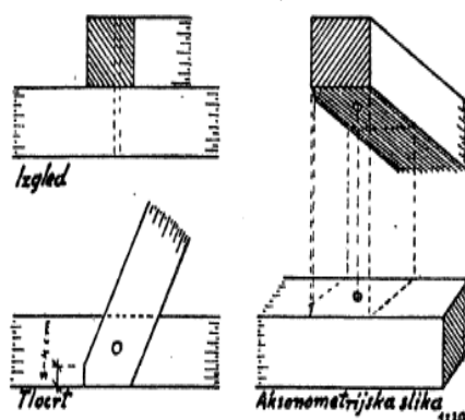
Slika 28. Jednostavno nalijeganje u horizontalnom kosom sudaranju [1]
