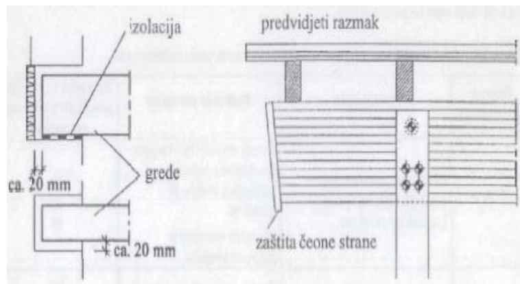
Slika 50. Ispravno naližganje grede na zid/beton (lijevo) te zaštita čeone strane glavnog nosača s prepustom (desno) [7]
