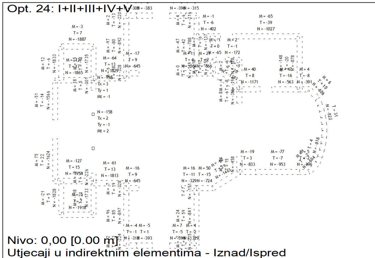
Slika 4.16. Prikaz opterećenja – kombinacija osnovnih opterećenja I+II+III+IV+V
