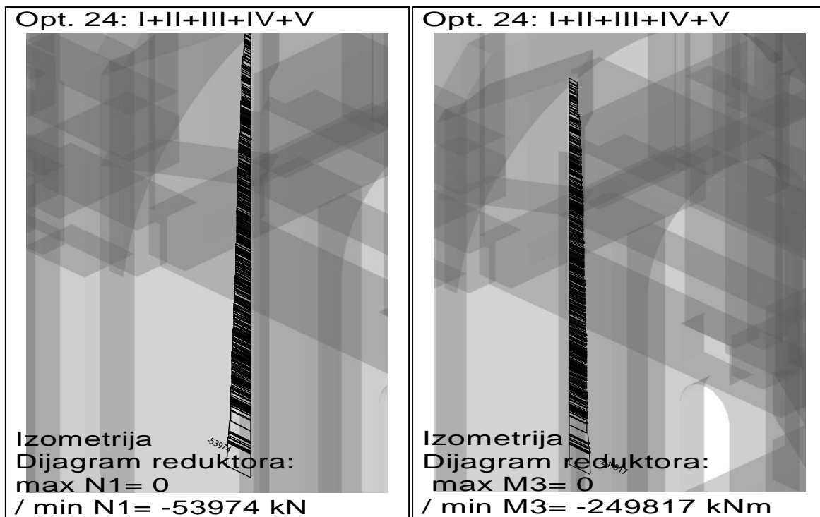
Slika 4.17. Prikaz najveće sile i najvećeg momenta - kombinacija osnovnih opterećenja I+II+III+IV+V
