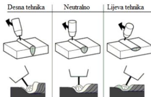
Slika 4.15 Tehnike zavarivanja [16]
