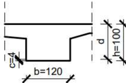
Slika 3.14. Određivanje statičke visine
