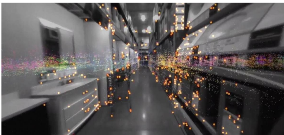
Slika 10: SLAM primjer
