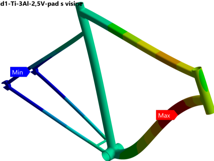
Prilog 22. Rezultati deformacija, naprezanja i pomaka FEA analiza VHybrid1 za Ti-3Al-2,5V slučaj pada s visine
