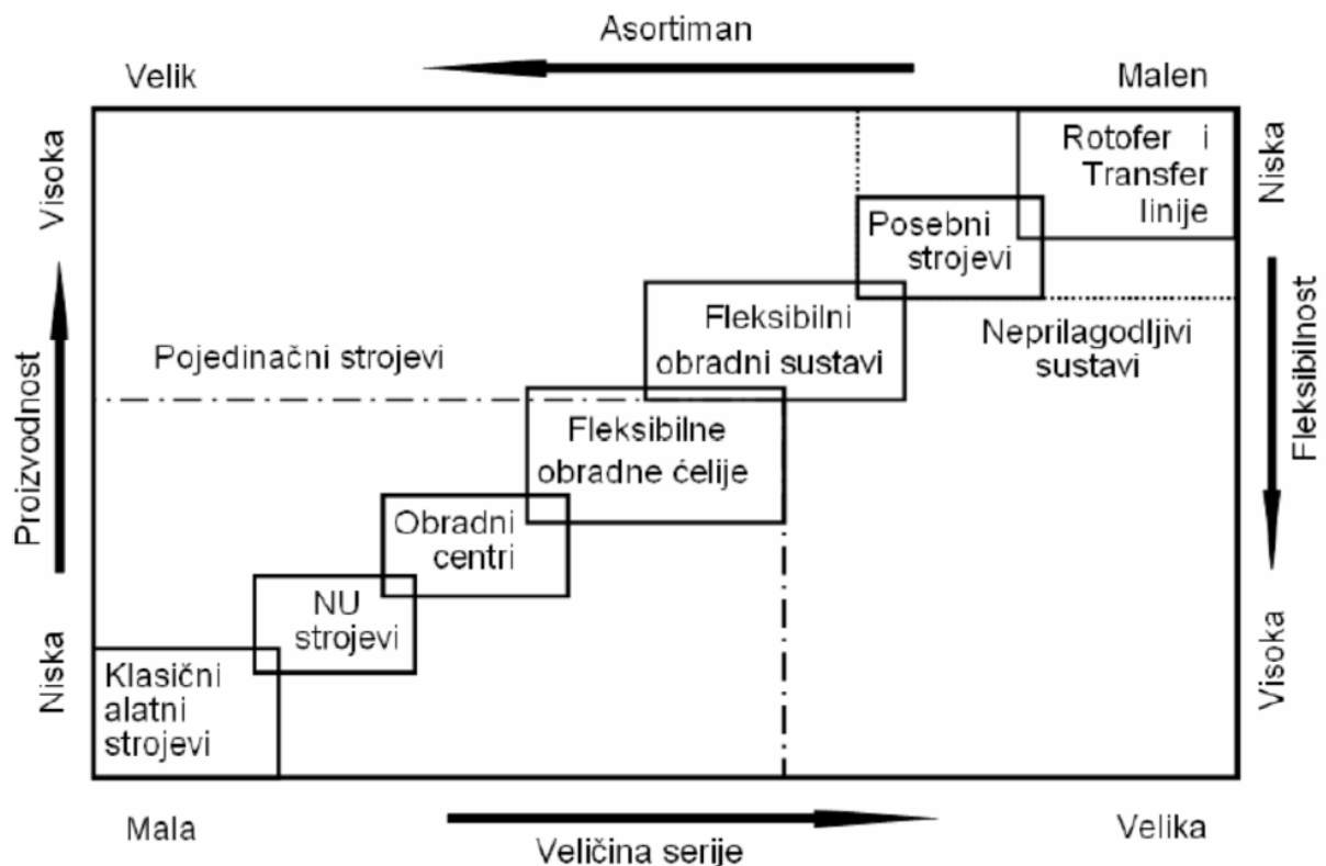
Slika 9. Podjela alatnih strojeva za glodanje prema tehnološkom prostoru [7]
