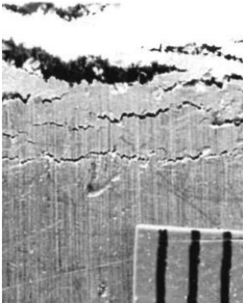
Slika 12 Interkristalna korozija Cr-Ni čelika [10]
