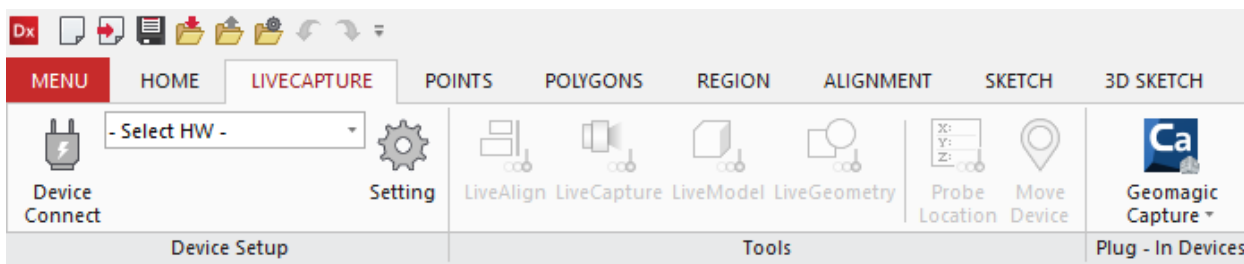
Slika 26 Livecapture tab
