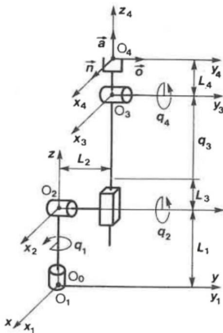
Slika 4 Vezani koordinatni sustav (u svrhu skice za izradu CAD modela)
