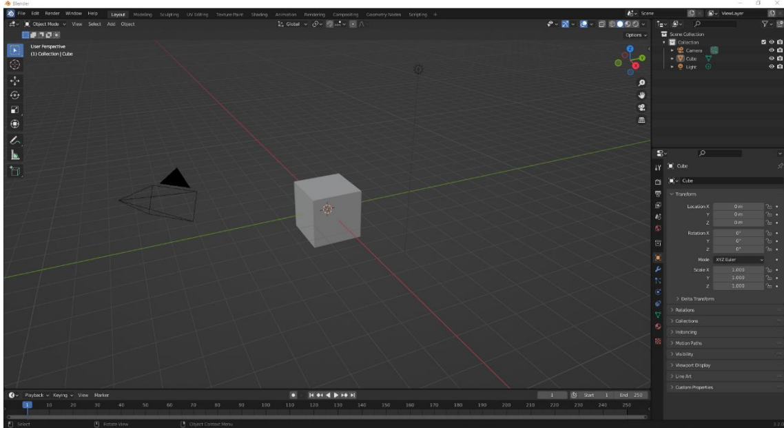
Slika 21 Blender program
