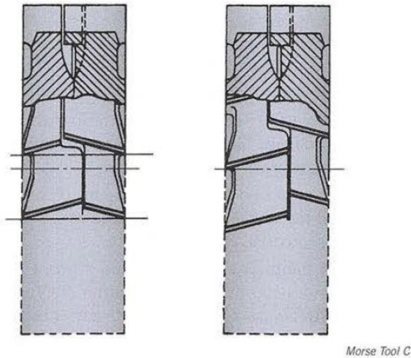
Slika 2.10 Rezne oštrice na isprepletenom koturastom glodalu [1]
