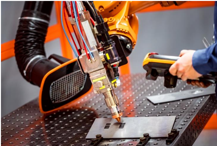
Slika 21. Plazma rezanje robotom [14]
