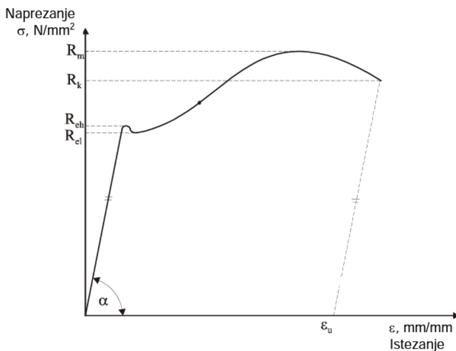
Slika 24. Konvencionalni dijagram naprezanje \sigma - istezanje \varepsilon [17]
