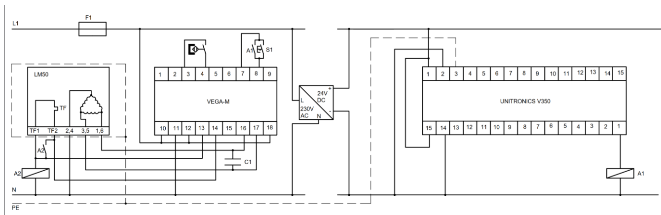
Slika 3.6.1. Električna shema
