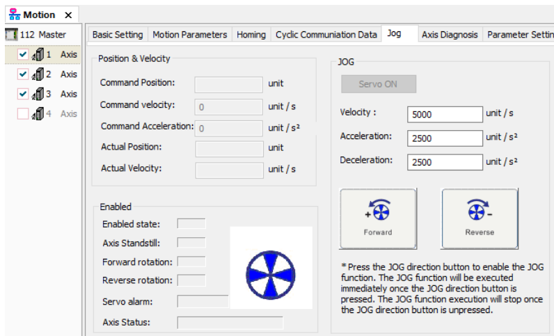
Slika 2.19 Prozor Jog u CANopen Builder programu [6]
