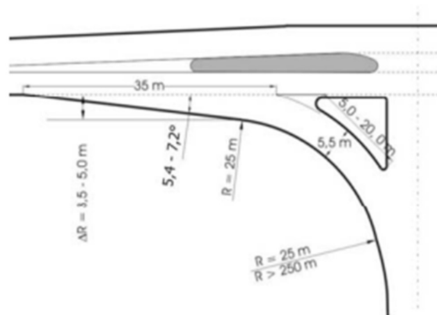
Slika 33. Izgradnja trake za skretanje desno na raskrižjima izvan urbanih područja [17]
