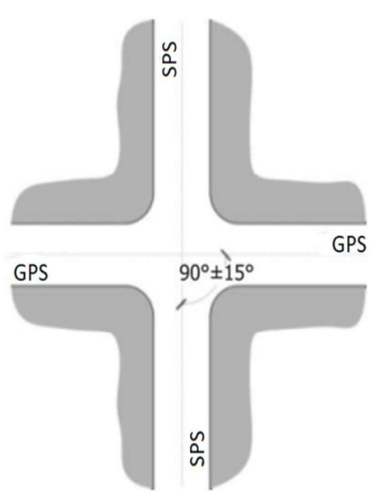
Slika 14. Četvorokrako raskrižje [17]
