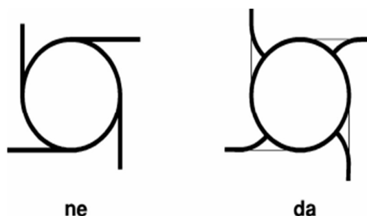
Slika 52. Pravač pružanja kraka kružnog raskrižja [17]
