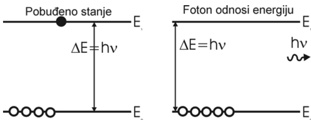
Slika 3. Spontana emisija [6]
