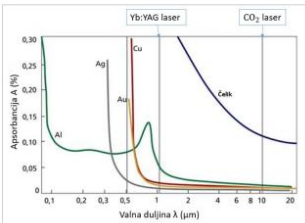
Slika 7 – Apsorbancija metala [9]
