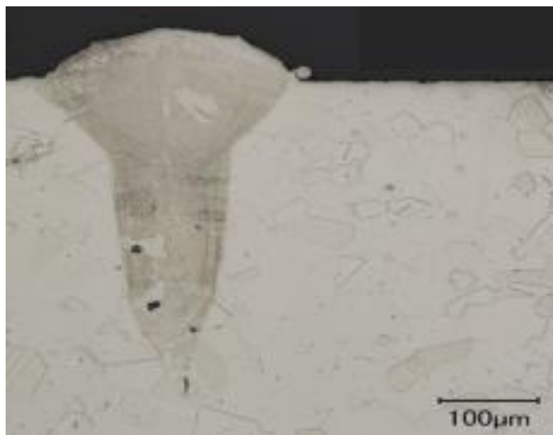
Slika 11 – Greške u mikrostrukтури tipa „Keyhole“ [7]
