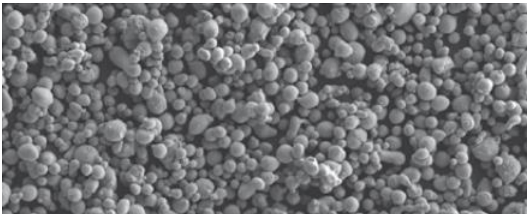
Slika 12 – Prah AlSi10Mg na SEM-u [13]
