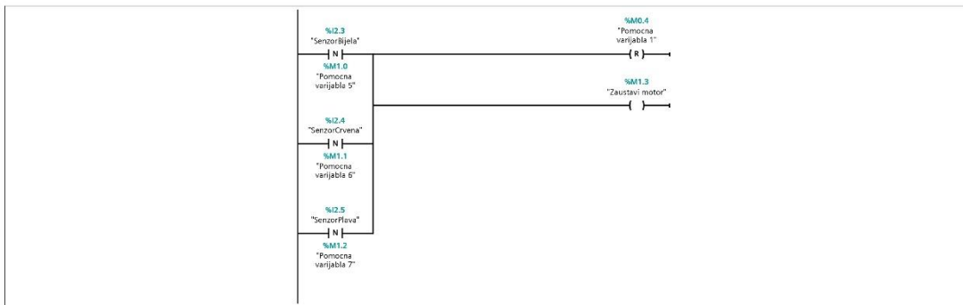
Network 10: Resetiranje pomocne varijable za brojac
