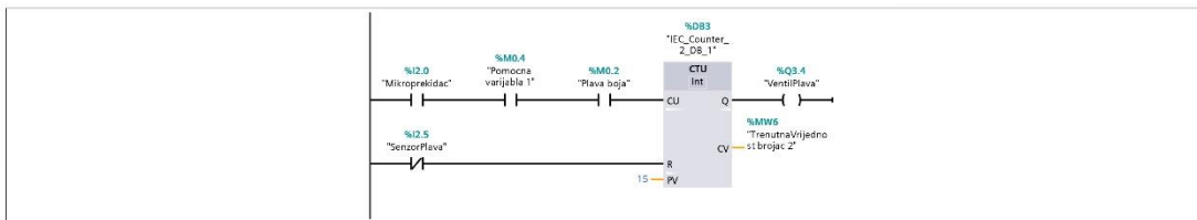
Network 9: Postavljanje pomocne varijable za brojac
