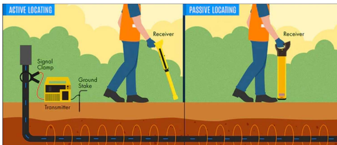
Slika 4.6: Prikaz razlike aktivnog i pasivnog lociranja vodova
