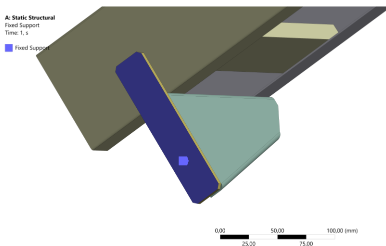
Slika 3.4 Fiksni oslonac
